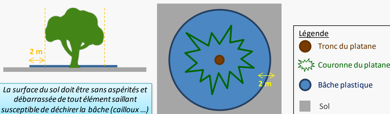
Fig. 14 - Disposition de la bache de protection au pied des platanes (gauche - vue de profil, droite - vue de dessus)
